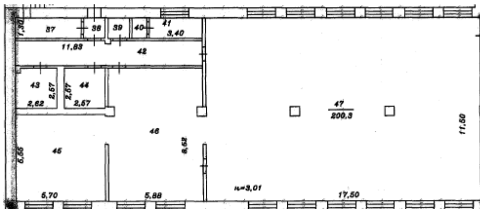
Рис.3. Столовая, пищеблок, первый этаж.
