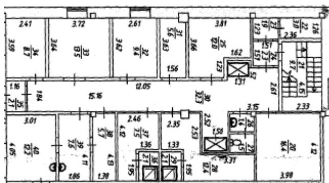
Рис 2. Пищеблок, цокольный этаж.
